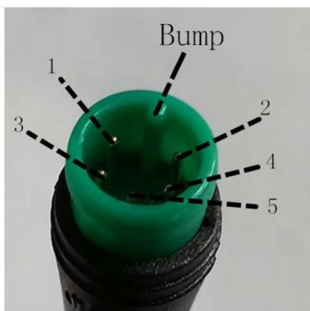
display end
